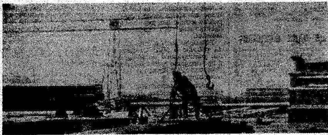
НА СНИМКАХ: идет укрупнительная сборка блоков девятого котла; слесарь-монтажник Василий Николаевич РОМАНОВ — один из ведущих звеньевых бригады В. С. Амеличева.
