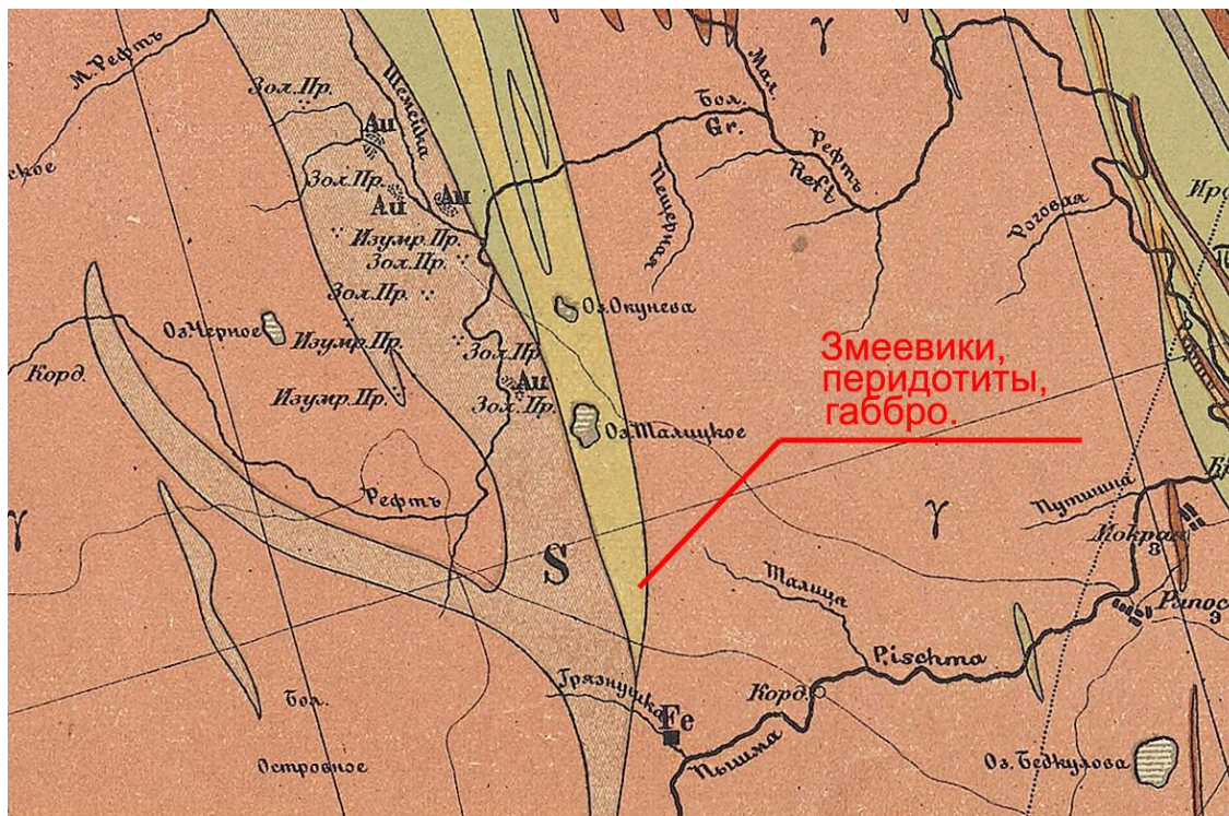
Фрагмент геологической карты Восточного склона Урала. Составитель: А. Карпинский - 1884 год.
